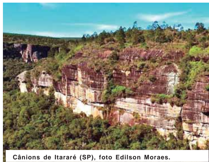
Cânions de Itararé (SP), foto Edilson Moraes.
